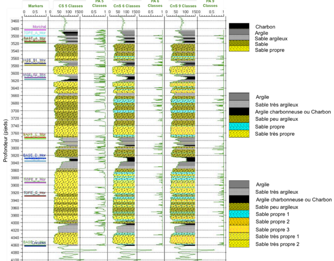
Figure 1.30 : Approches supervisée (CS 5) vs. non supervisées (Cns 6 et Cns 9) des électrofaciès pour le puits A.
