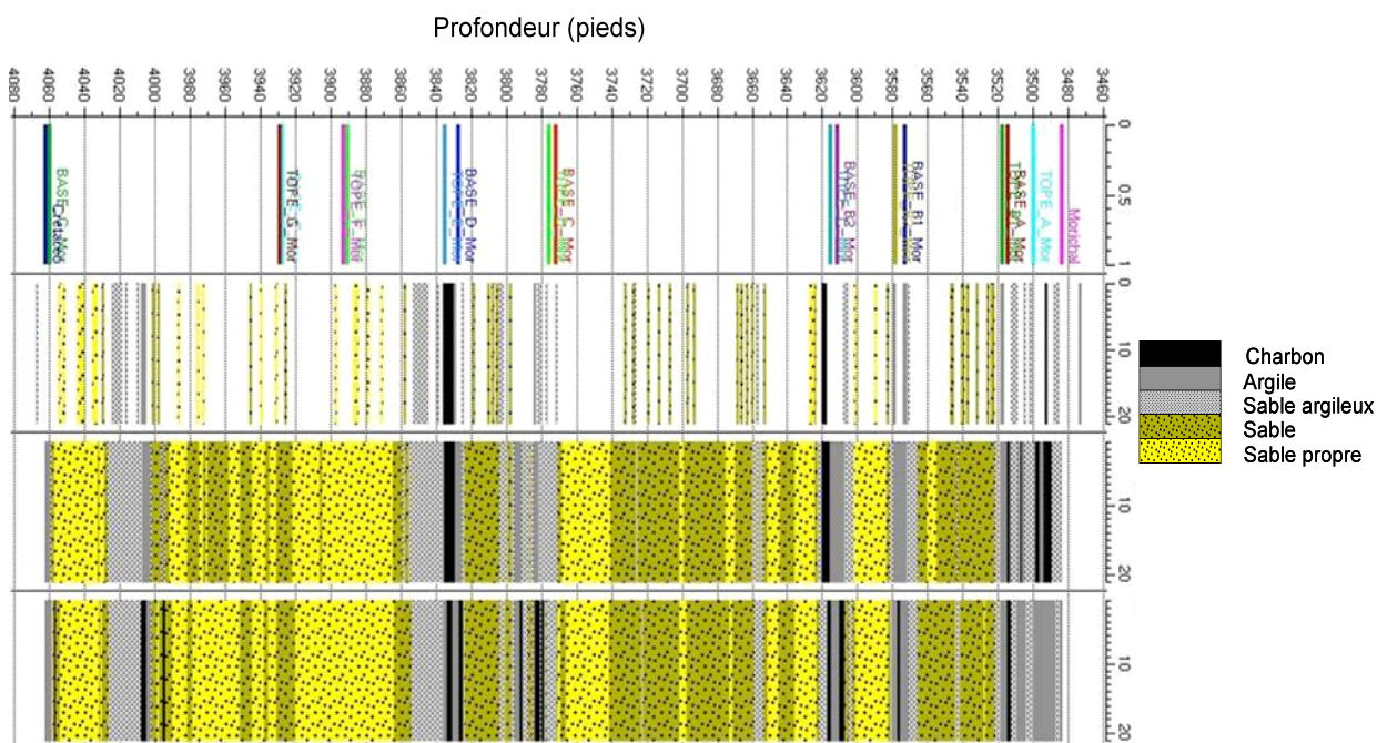
Figure 6.5 : Puits A : carotte interprétée (en haut), diagraphie électrofaciès générée à partir des diagraphies Gamma Ray (GR), Porosité-Neutron (NPHI), Résistivité (RD) et Densité (RHOB) (au milieu), nouvelle diagraphie électrofaciès générée à partir des diagraphies porosité \phi , volume d'argile V_{sh} et saturation en eau S_w (en bas).
