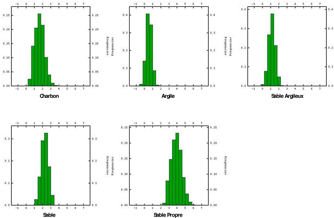
Figure 7.6 : Distribution du \log(RD) (ohm-m) simulé par faciès dans la séquence A-B.
