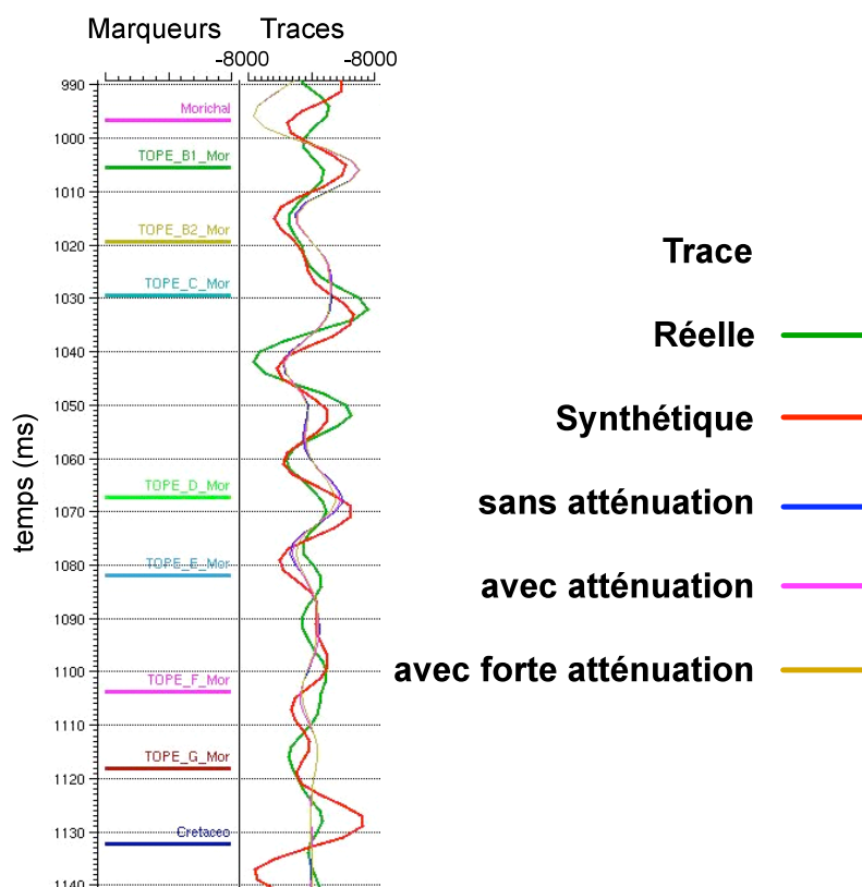
Figure 10.10 : Comparaison de la trace sismique réelle optimale (verte), de la trace synthétique optimale finale (rouge), des traces sans atténuation (bleue), avec atténuation sur le réservoir (fuchsia) et avec forte atténuation sur le réservoir (ocre) issues de la modélisation 1D, pour le stack total .
