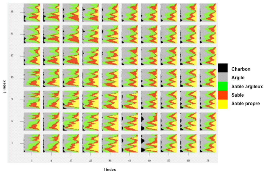
Figure 6.10 : MPV de la séquence A-B.
