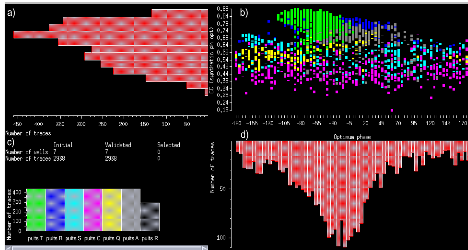
Figure 4.11 : Estimation de la phase de l'ondelette pour le stack total : a) Histogramme du coefficient de corrélation entre trace synthétique et trace réelle, b) Diagramme croisé « phase vs coefficient de corrélation », c) Puits utilisés et d) Histogramme de la phase optimale déterminée aux différentes traces.
