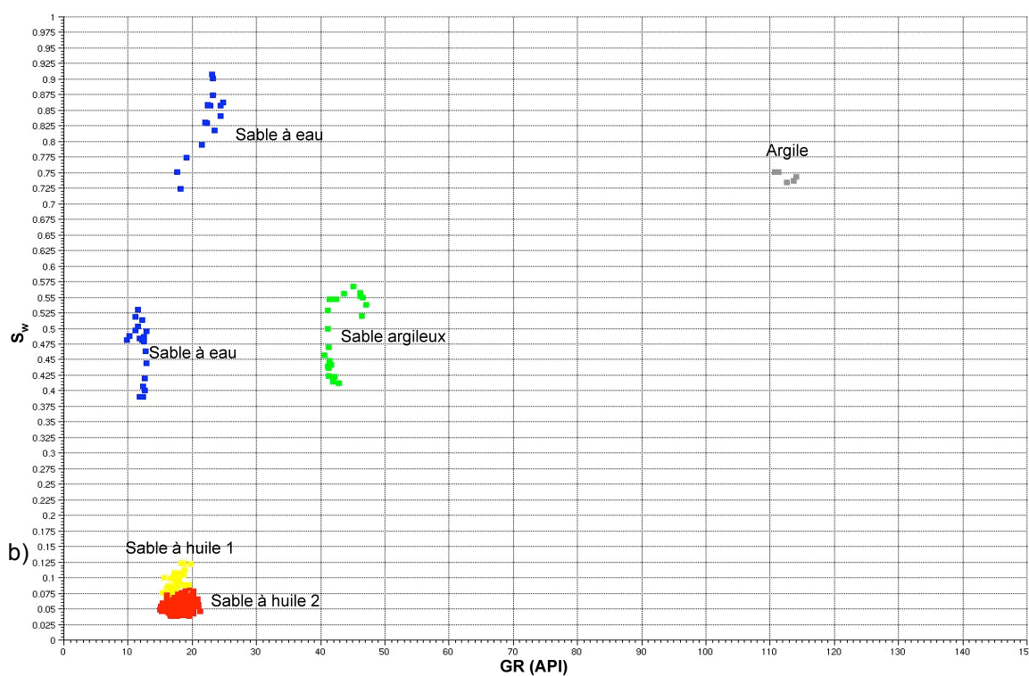
Figure 1.35 : Diagramme croisé entre : a) la porosité et l'impédance et b) le Gamma-Ray et la saturation en eau ( S_w ), pour les échantillons des pics de la fonction de densité de probabilité déroulée.
