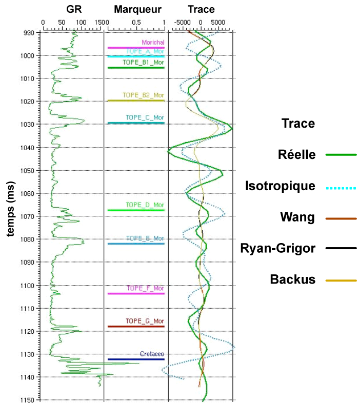
Figure 9.10 : Comparaison des traces : sismique réelle optimale (verte), synthétique isotrope (pointillé cyan) et anisotropes par les modèles de Wang (marron), Ryan-Grigor (noire) et Backus (ocre) pour le stack Total au puits A.
