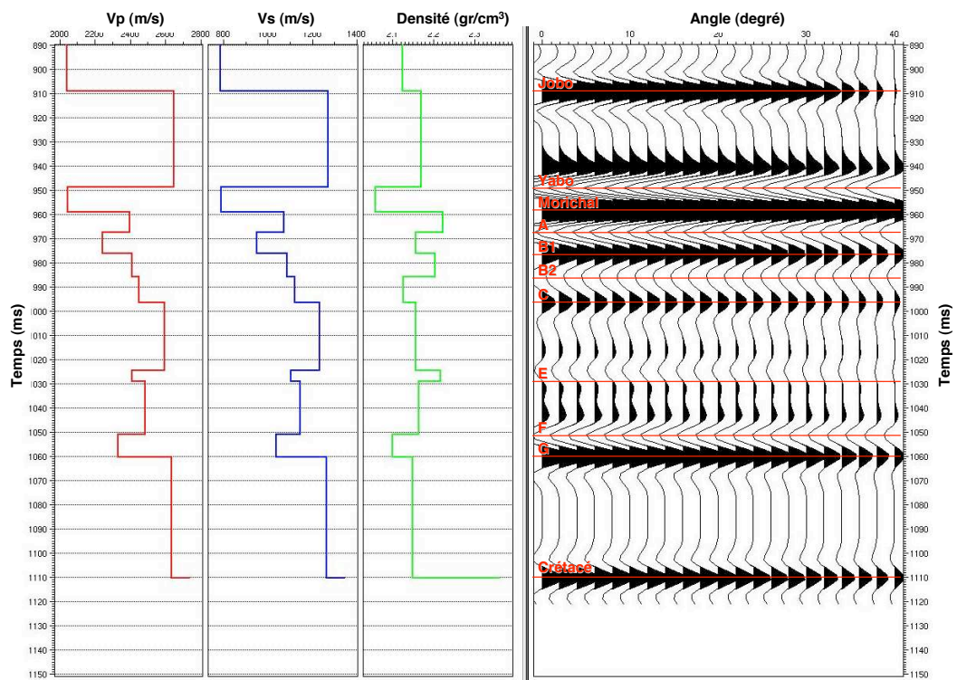
Figure 3.3 : Modélisation AVO (sismogramme synthétique) des puits A (au-dessus), B (centre) et C (au dessous) avec les valeurs moyennes par intervalles de V_p , V_s et Densité. Les valeurs des amplitudes sont comprises entre -0,5 et 0,5.
