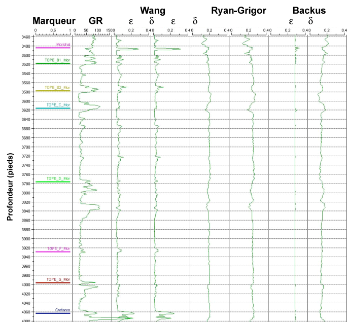
Figure 9.6 : Diagraphies de \delta et \epsilon pour chaque modèle Wang, Ryan-Grigor et Backus dans les puits A.
