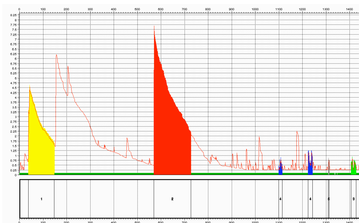
Figure 1.33 : Choix de 5 classes sur la fonction de densité déroulée, et échantillons d'apprentissage associés (en couleur).
