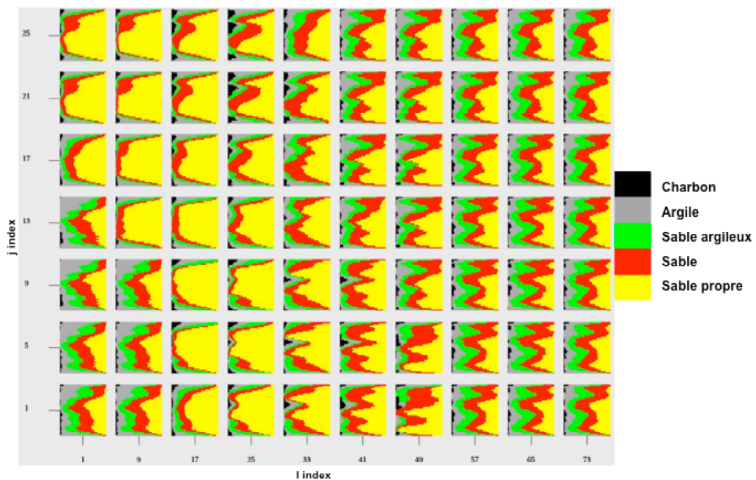
Figure 6.11 : MPV de la séquence C.
