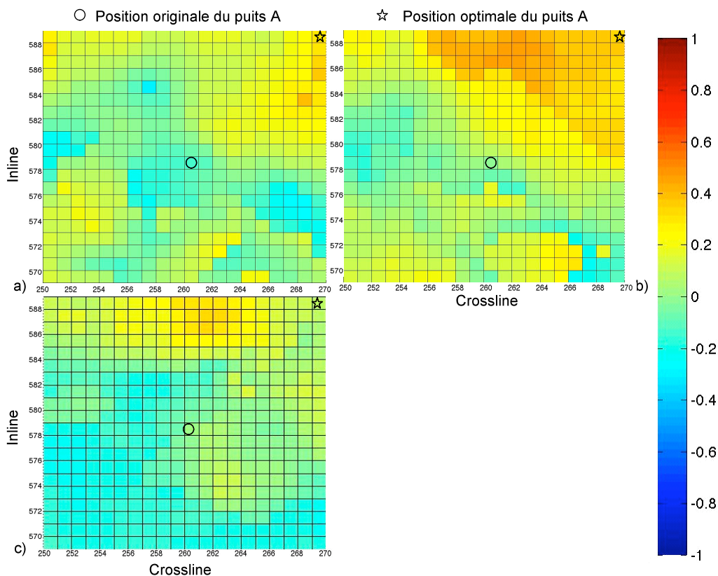
Figure 10.12 : Carte du coefficient de corrélation dans un mini-cube de 21 x 21 traces autour du puits A (indiqué par un cercle) de la sismique de la classe d'angles 24^{\circ} - 36^{\circ} et les traces : a) la trace isotrope optimale finale , b) la trace isotrope zéro-phase et c) la trace viscoélastique 1D sans atténuation dans le réservoir Morichal. La position optimale du calage isotrope est indiquée par une étoile.
