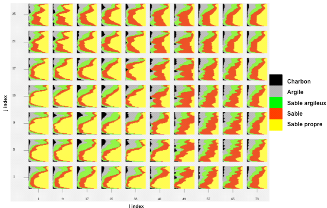
Figure 6.12 : MPV de la séquence D-E.
